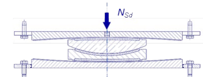
2 a) Normalzustand
