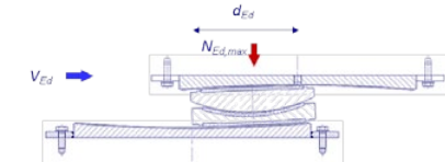
2 b) Erdbebenfall
