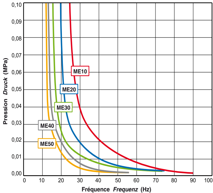
GRAPHIQUE FRÉQUENCE PROPRE DU MEGAMAT BASSE DENSITÉ GRAFIK DER EIGENFREQUENZ VON MEGAMAT MIT NIEDRIGER DICHTE
