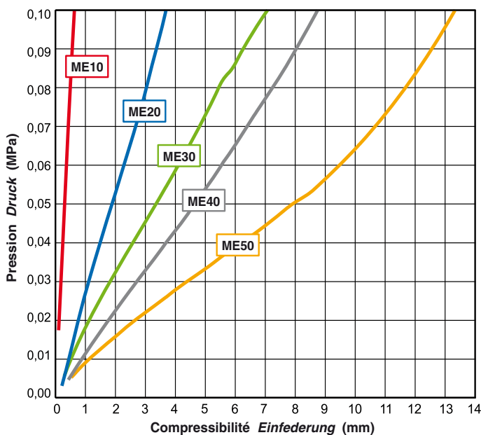
GRAPHIQUE DE CHARGE - DÉFORMATION DU MEGAMAT BASSE DENSITÉ EINFEDERUNGSGRAFIK BEI NIEDRIGER DICHTE
