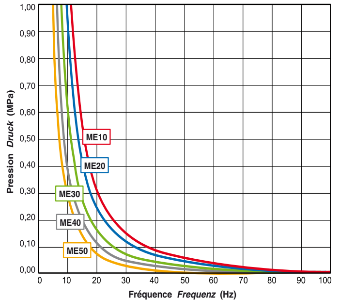
GRAPHIQUE FRÉQUENCE PROPRE DU MEGAMAT HAUTE DENSITÉ GRAFIK DER EIGENFREQUENZ VON MEGAMAT MIT HOHER DICHTE
