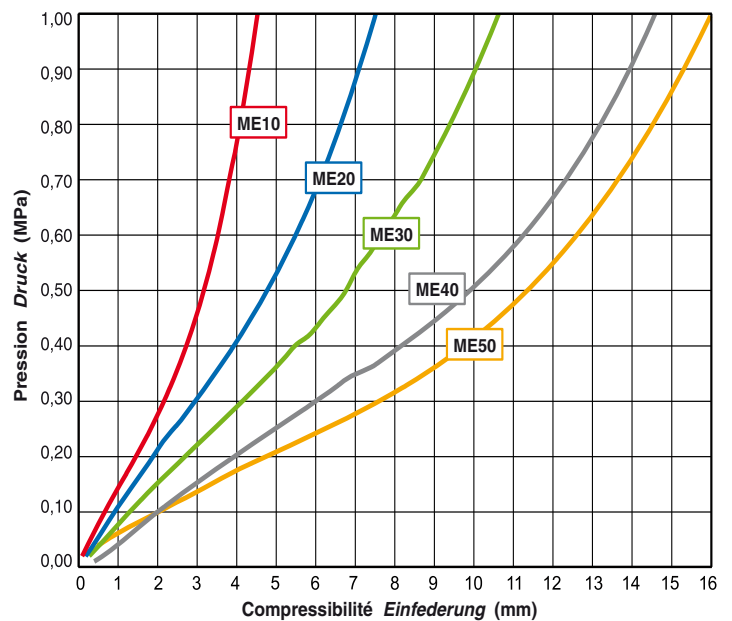
GRAPHIQUE DE CHARGE - DÉFORMATION DU MEGAMAT HAUTE DENSITÉ EINFEDERUNGSGRAFIK BEI HOHER DICHTE
